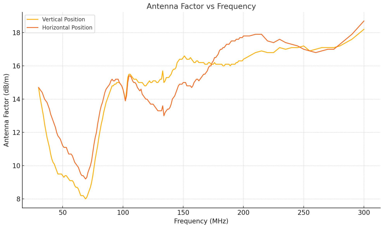
天线因子图
