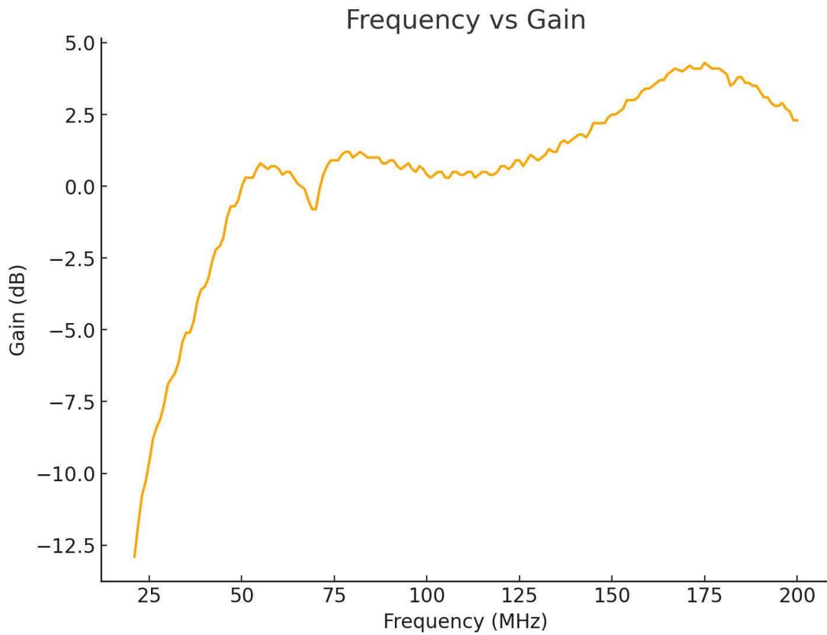
天线增益图
