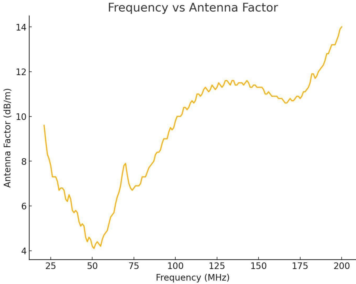
天线系数图
