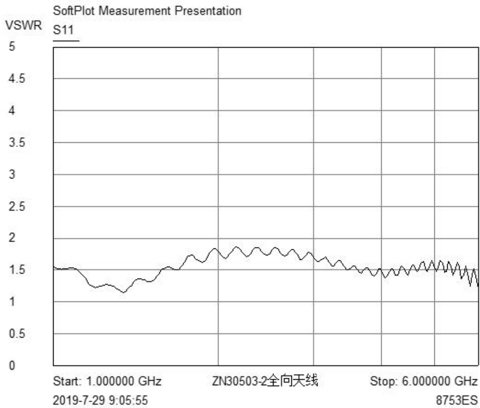
驻波图
