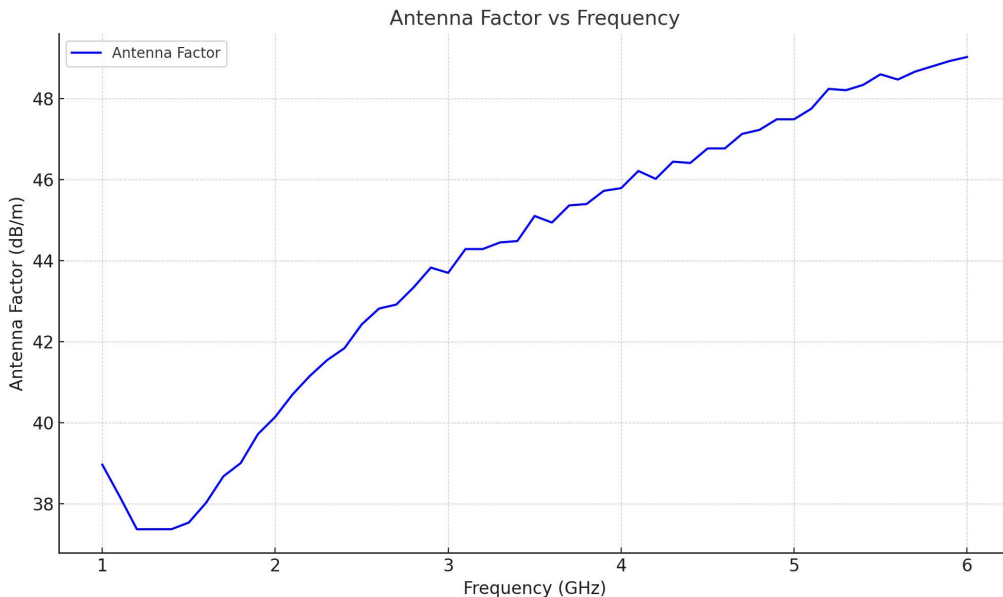
天线因子图
