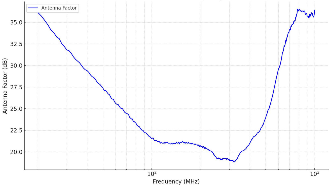
天线系数图
