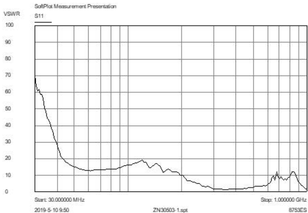
天线驻波
